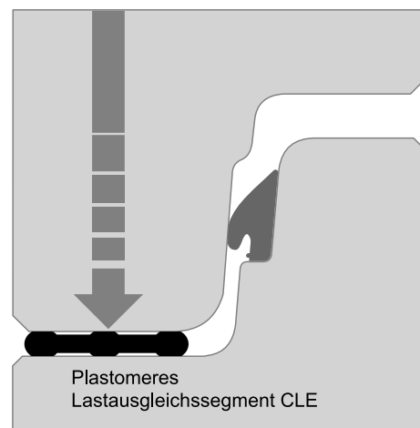
CLE ist mit verschiedenen Dichtungen einsetzbar (Beispiel: SD-97)
